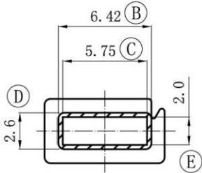
A-A SECTION
